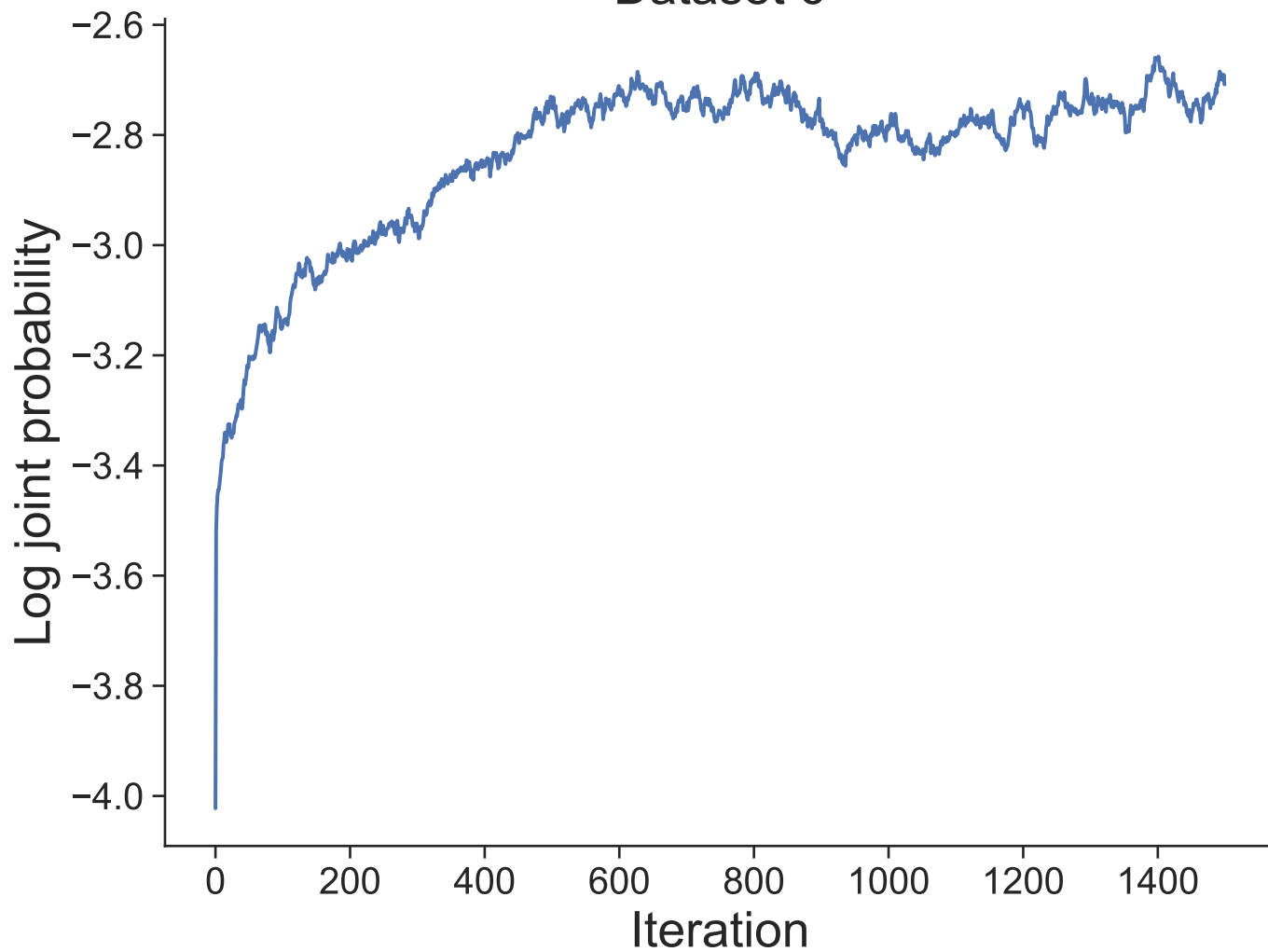
Dataset 6
