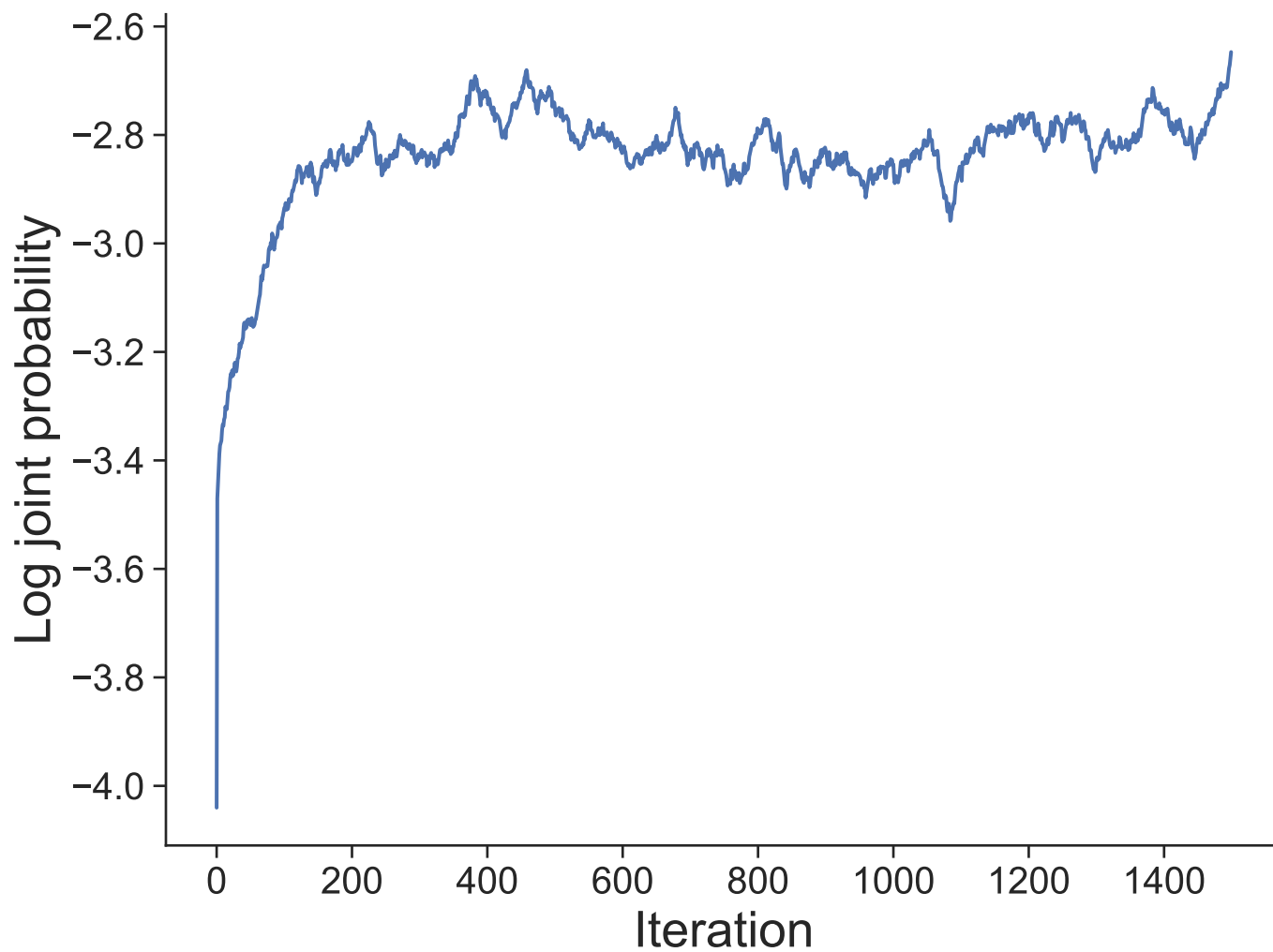
Dataset 22
