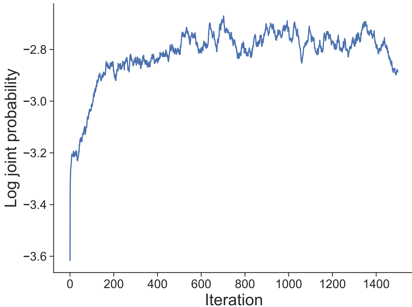
Dataset 0
