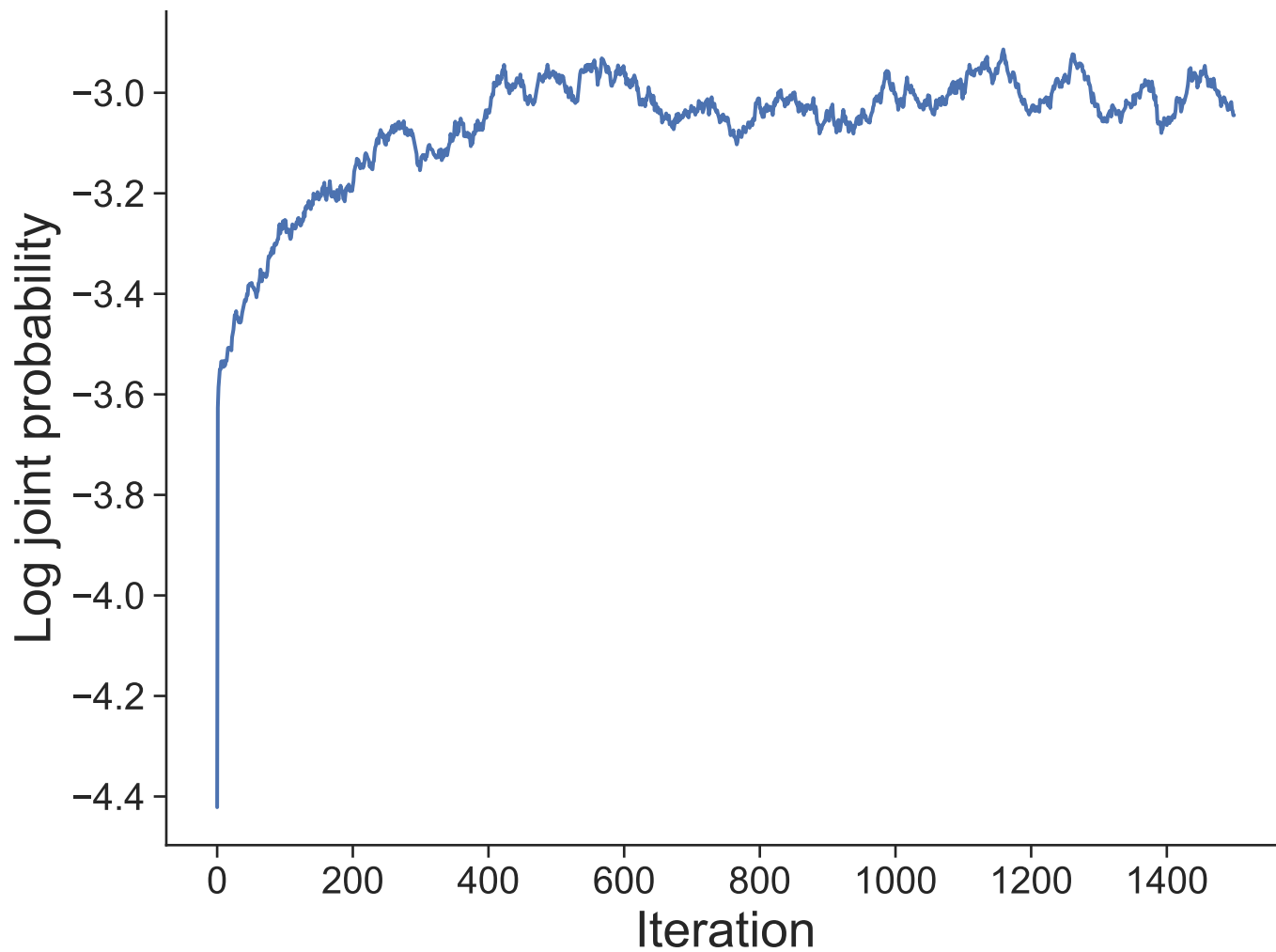
Dataset 3
