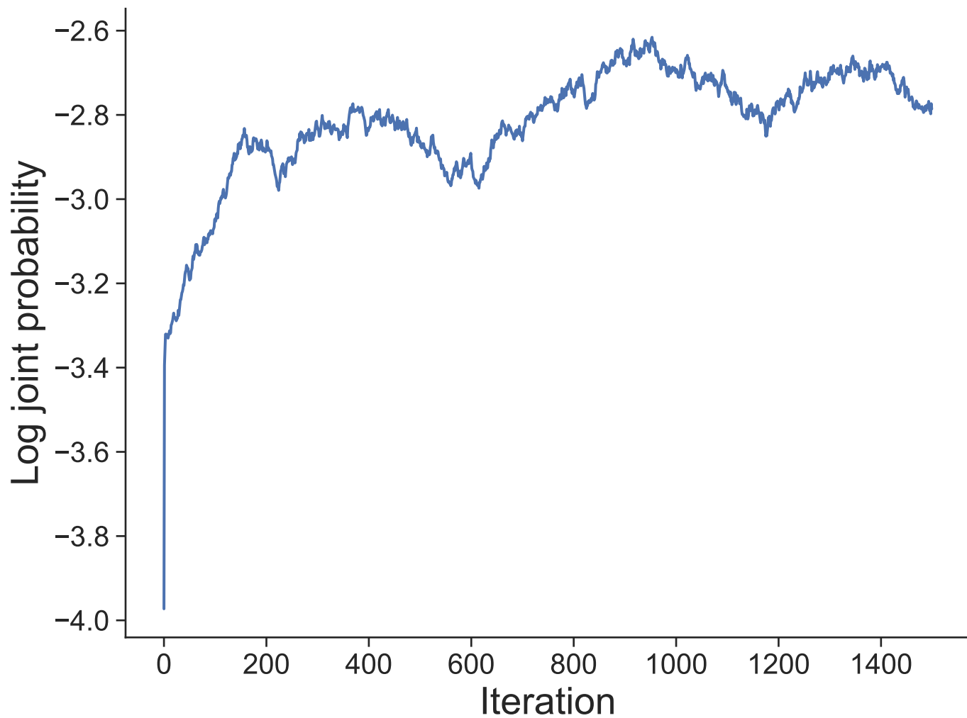
Dataset 2
